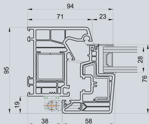
Telaio a L + anta ridotta
