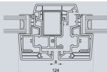
Nodo Centrale Simmetrico
