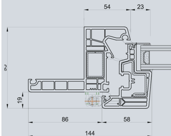
Telaio a Z65 + anta ridotta
