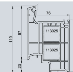
Zoccolo a scatto
