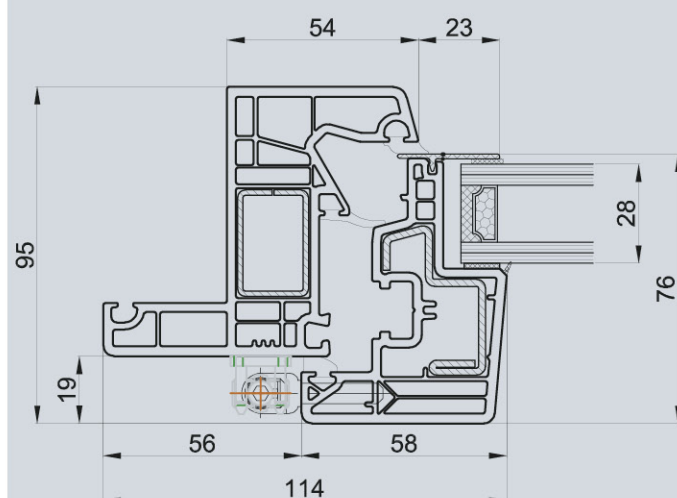
Telaio a Z35 + anta ridotta
