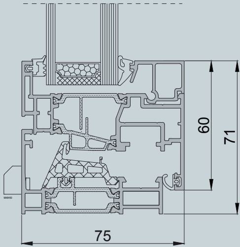
Telaio a L stretto + anta
