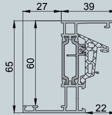
Telaio Z27 stretto
