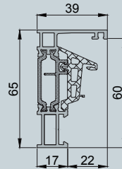
Telaio L stretto
